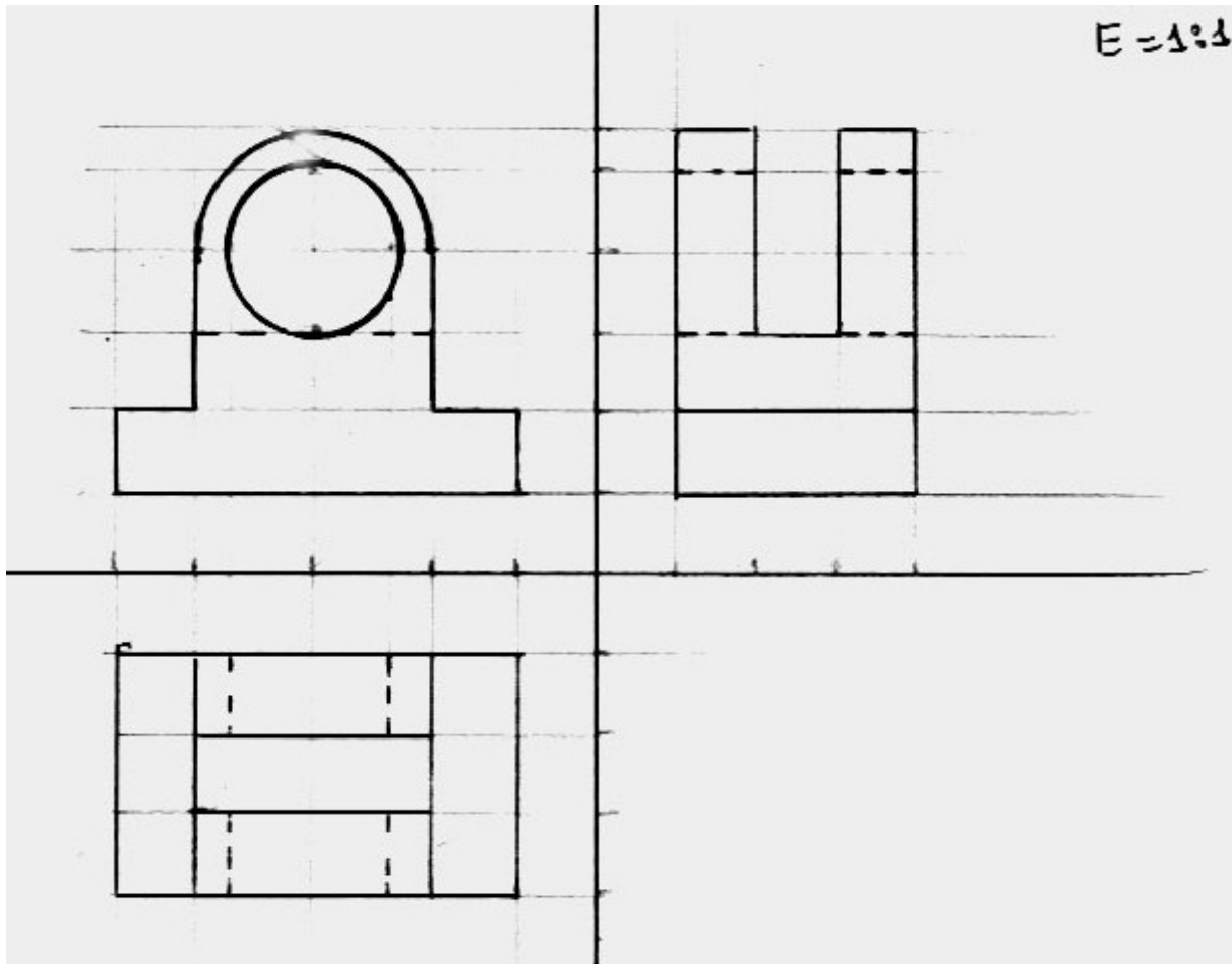
PIEZA F.
