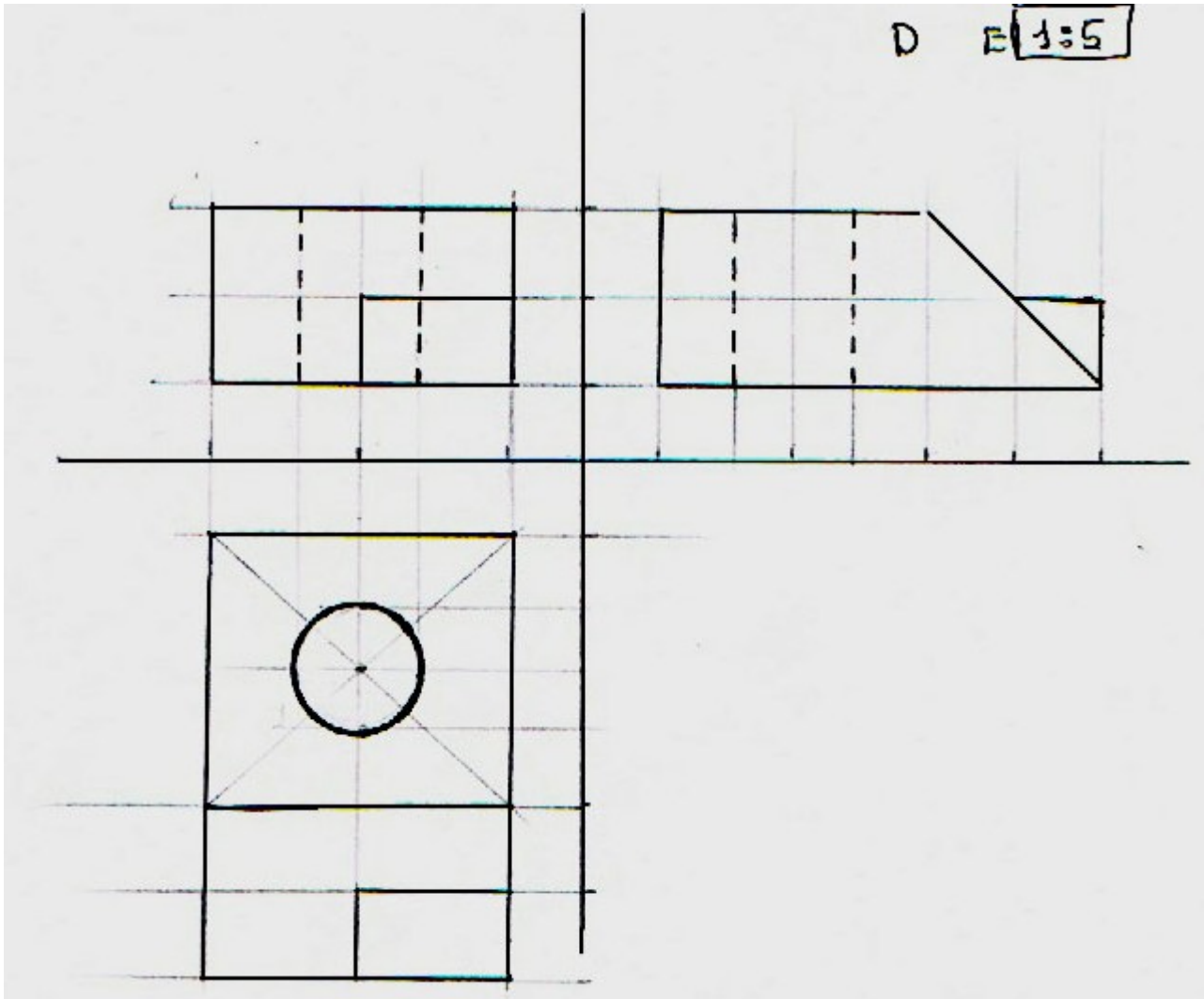
PIEZA D
