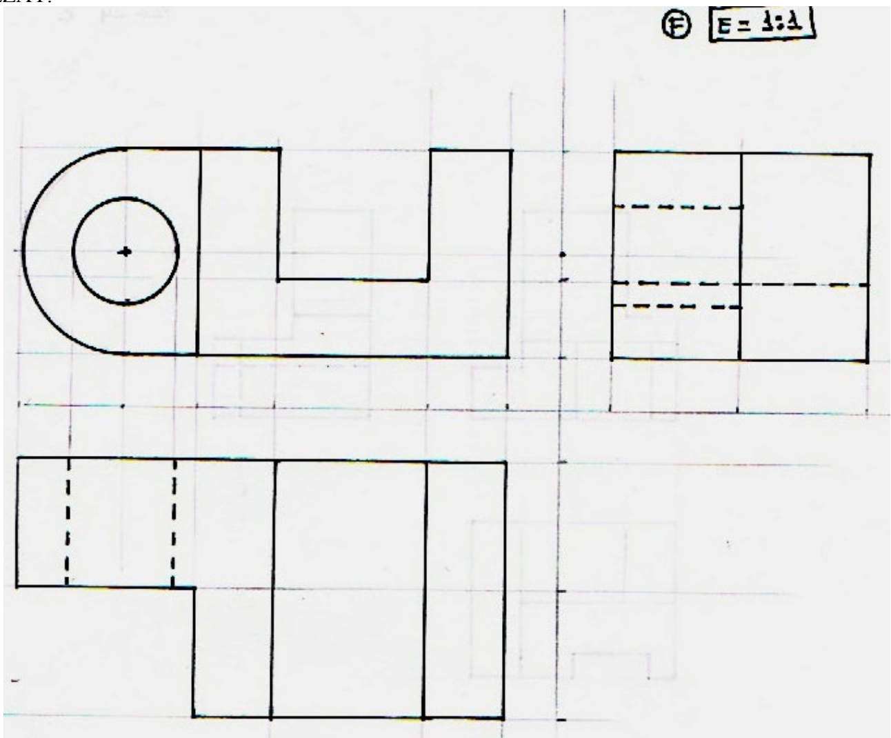
PIEZA F.
