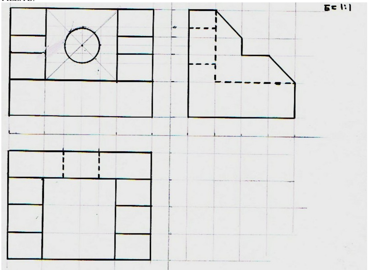
PIEZA B.
